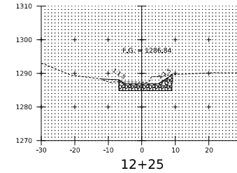
12+25
