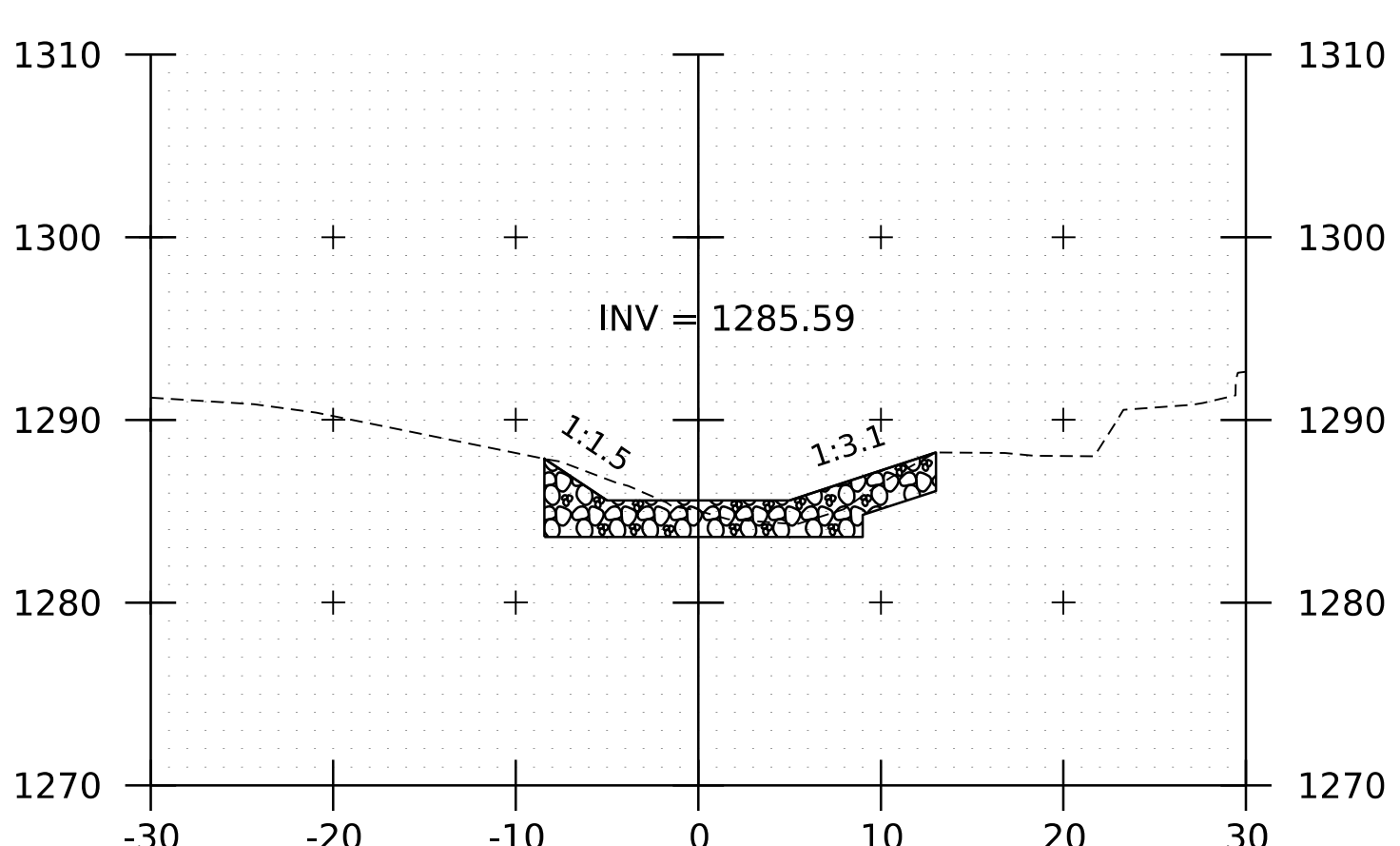
11+00
