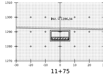
11+75
