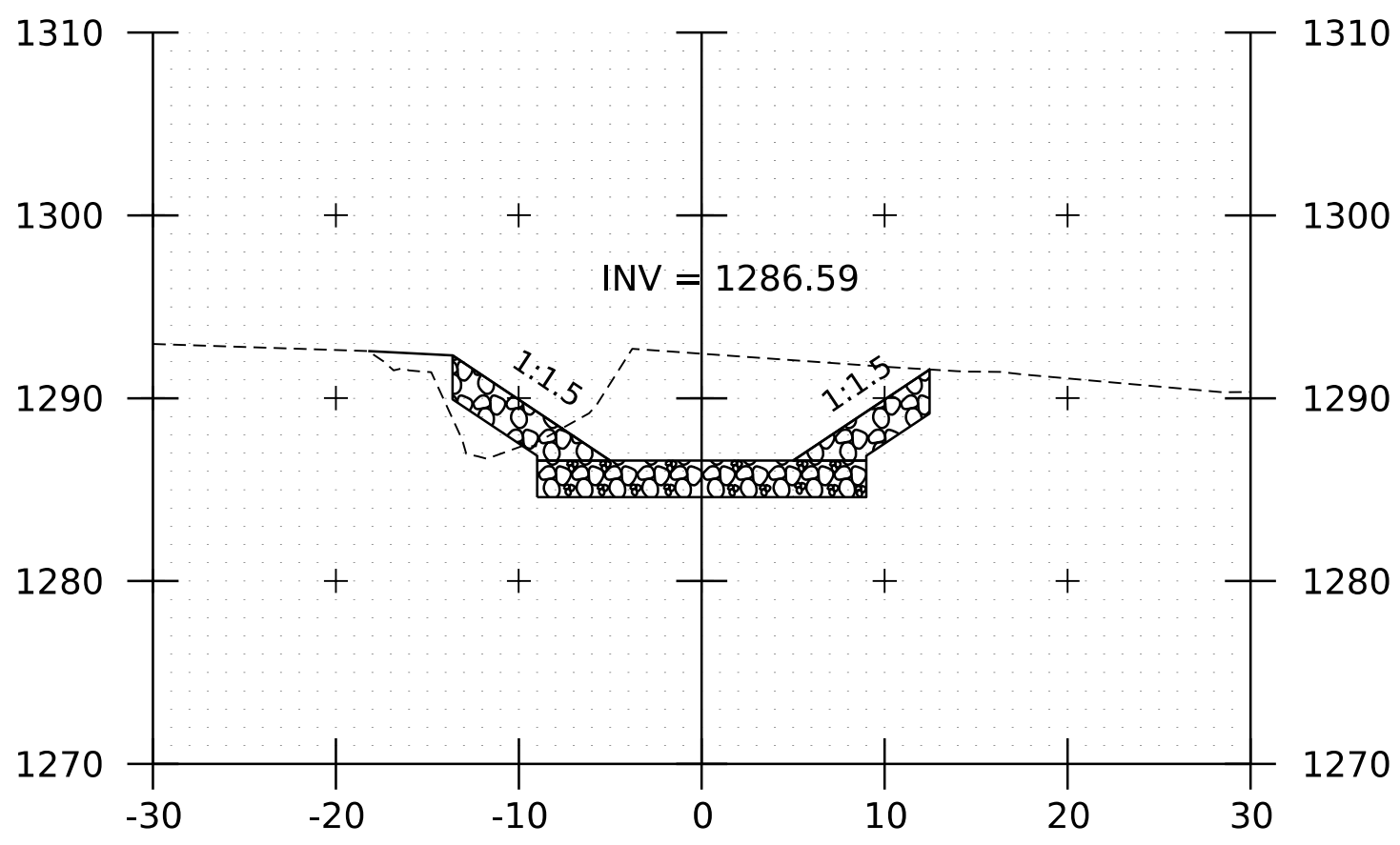
12+00
