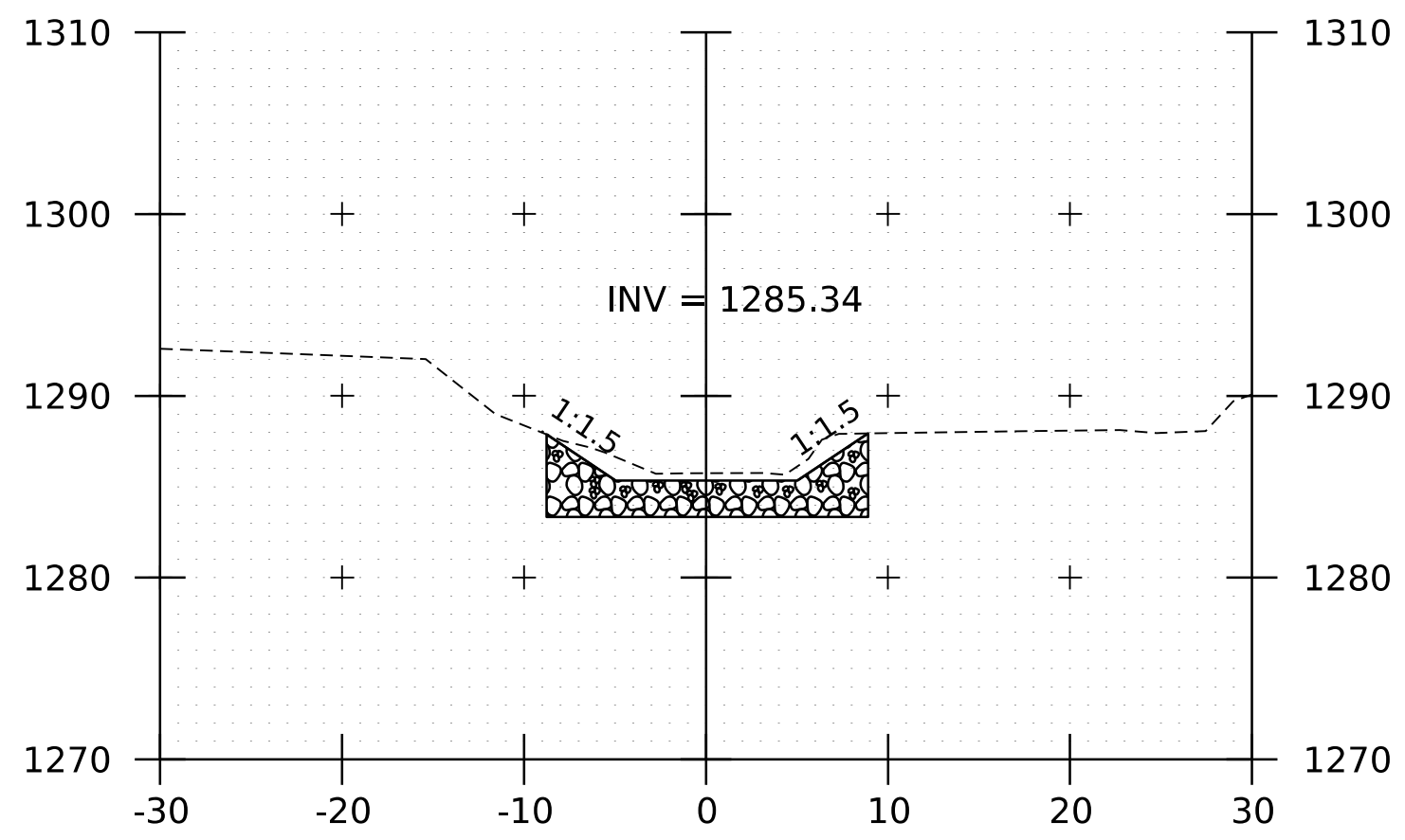
10+75
