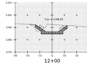
12+00
