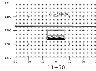
11+50
