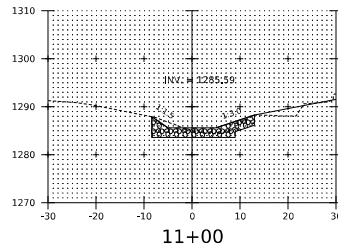
11+00
