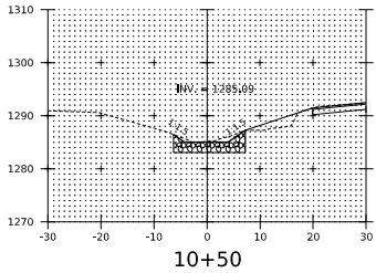
10+50
