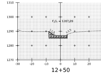
12+50
