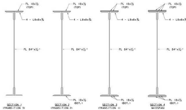
GIRDER SECTIONS SCALE: 1" = 1'-0"
